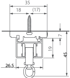
* 1: レール幅寸法 * 2: レール高さ寸法
