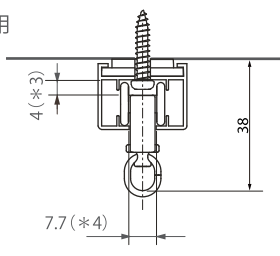
* 3: ネジ頭クリアランス * 4: レール開口幅
