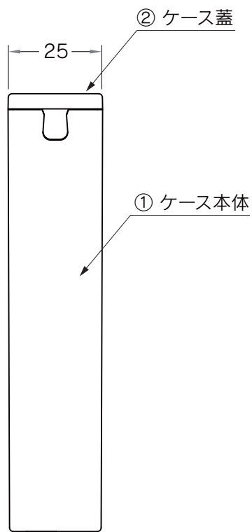
[側面図]
